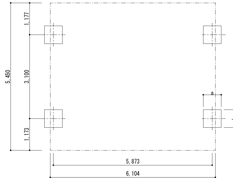
■基礎配置図
